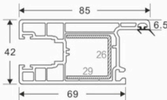
85 SLIDING DOOR SASH 2 CODE : SB-1005
