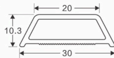
30 MM D-STRIP CODE : SB-D1
