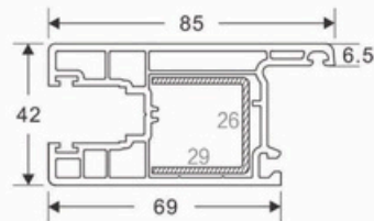
B5 SLIDING DOOR SASH 2 CODE : SB-1005
