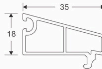
60 OUT WARD DOOR SASH CODE : SB-3003
