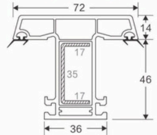
60 MULLION CASEMENT CODE : SB-3004
