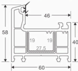
60 CASEMENT OUTER FRAME CODE : SB-3001
